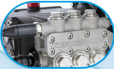
Pompa Alta Pressione (6000 ore prima manutenzione)
